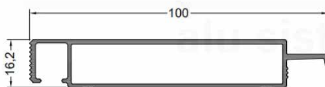
ALB4-934 PREMARCO Peso: 0,900 kg/m 5T por Paquete
