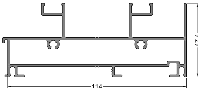
ALB4-263 UMBRAL/DINTEL DE MARCO Peso: 1,857 kg/m 2T por Paquete
