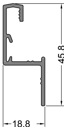
ALB4-264 GUÍA CORREDIZA MOSQUITERO Peso: 0,350 kg/m 10T por Paquete
