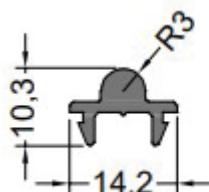
ALB4-059 CORREDIZA GUÍA CON RADIO 3MM Peso: 0,152 kg/m 10T por Paquete
