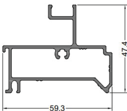
ALB4-283 ACOPLE UMBRAL/DINTEL Peso: 0,924 kg/m 2T por Paquete
