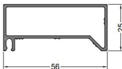
ALB4-284 ACOPLE JAMBA DE MARCO Peso: 0,639 kg/m 2T por Paquete
