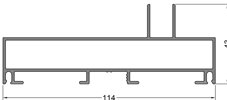
ALB4-262 JAMBA DE MARCO Peso: 1,351 kg/m 2T por Paquete
