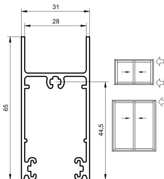
ALB3-073 ZÓCALO Y CABEZAL CORREDIZA P/DVH (0,861 Kg/m) Tiras por Paquete 4
