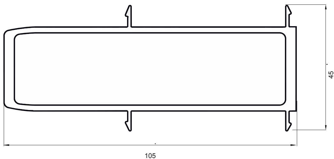
ALB3-068 ACOPLE REFORZADO PAÑO FIJO (1,758 Kg/m) Tiras por Paquete 2
