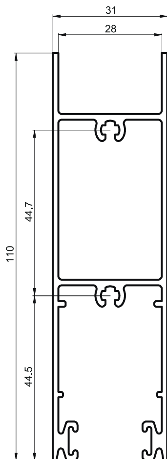
ALB3-074 ZÓCALO ALTO CORREDIZA P/DVH (1,412 Kg/m) Tiras por Paquete 2
