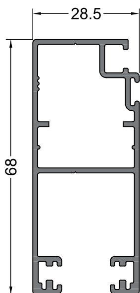
ALB4-062 PERFIL DE MOSQUITERO Peso: 0,888 kg/m 4T por paquete
