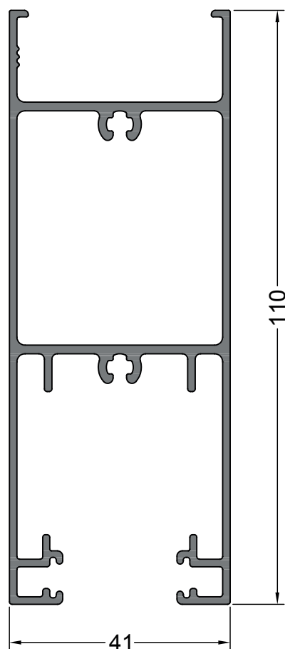
ALB4-260 ZÓCALO ALTO CORREDIZA DVH Peso: 1,537 kg/m 2T por paquete
