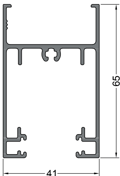
ALB4-261 ZÓCALO CABEZAL CORREDIZA DVH Peso: 0,955 kg/m 3T por paquete
