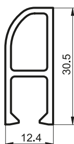
ALB3-039 TOPE MOSQUITERO (0,329 Kg/m) Tiras por Paquete 10
