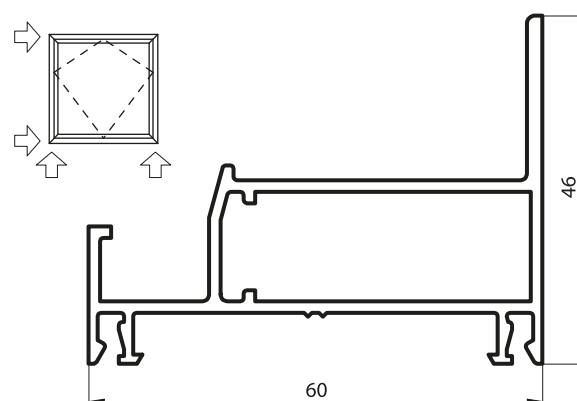
ALB3-057 MARCO VENTANA DESPLAZABLE (0,837 Kg/m) Tiras por Paquete 4
