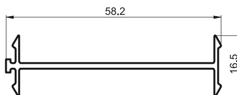
ALB3-067 PERFIL DE ACOPLE (0,329 Kg/m) Tiras por Paquete 10
