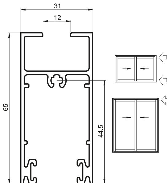
ALB3-061 ZÓCALO Y CABEZAL VENTANA CORREDIZA (0,942 Kg/m) Tiras por Paquete 4
