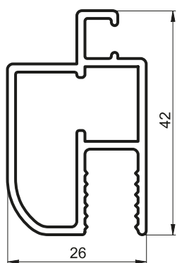
ALB3-038 MOSQUITERO REFORZADO (0,594 Kg/m) Tiras por Paquete 2
