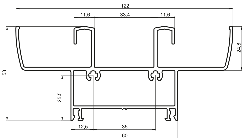
ALB3-037 UMBRAL Y DINTEL DE MARCO (1,744 Kg/m) Tiras por Paquete 2
