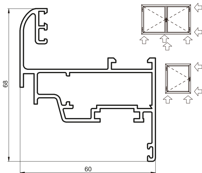
ALB3-052 HOJA CURVA VENTANA DE ABRIR (1,139 Kg/m) Tiras por Paquete 2
