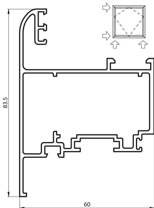
ALB3-056 HOJA CURVA VENTANA DESPLAZABLE (1,337 Kg/m) Tiras por Paquete 2
