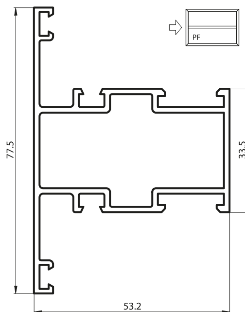
ALB3-060 TRAVESAÑO PAÑO FIJO (1,091 Kg/m) Tiras por Paquete 3
