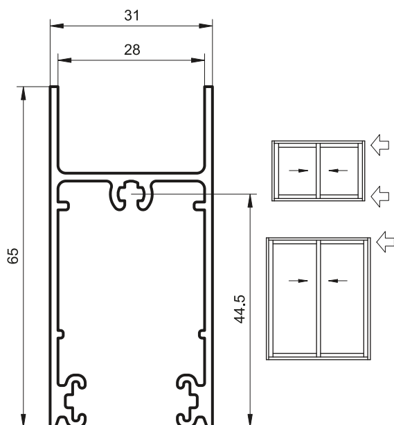
ALB3-073 ZÓCALO Y CABEZAL CORREDIZA P/DVH (0,861 Kg/m) Tiras por Paquete 4
