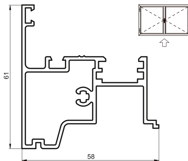
ALB3-053 ENCUENTRO CENTRAL VENTANA DE ABRIR (1,094 Kg/m) Tiras por Paquete 2
