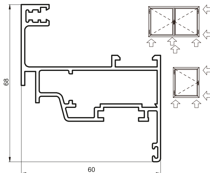
ALB3-054 HOJA RECTA VENTANA DE ABRIR (1,148 Kg/m) Tiras por Paquete 2
