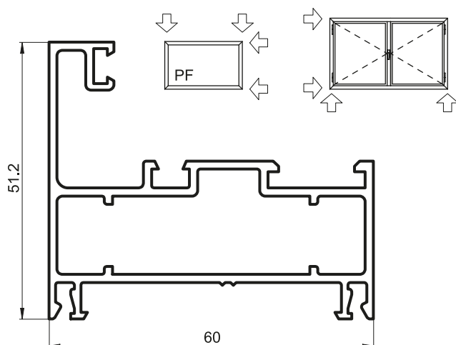
ALB3-059 MARCO RECTO PAÑO FIJO Y VENTANA DE ABRIR (1,053 Kg/m) Tiras por Paquete 2
