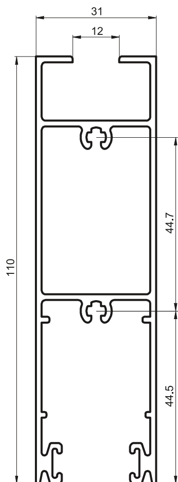
ALB3-062 ZÓCALO ALTO PUERTA CORREDIZA (1,477 Kg/m) Tiras por Paquete 2
