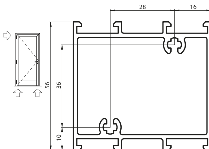
ALB3-042 TRAVESAÑO PUERTA DE REBATIR (1,399 Kg/m) Tiras por Paquete 2
