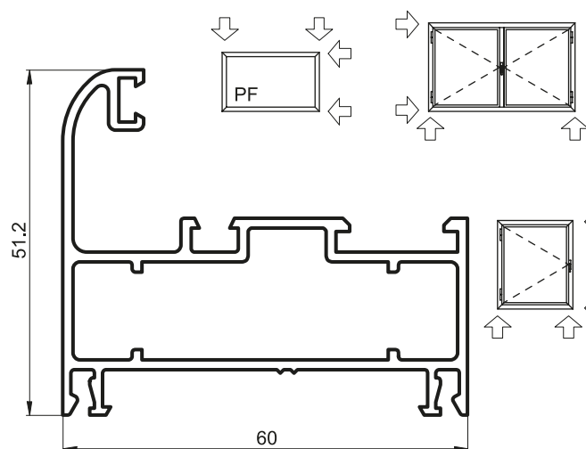
ALB3-055 MARCO PAÑO FIJO Y VENTANA DE ABRIR (1,037 Kg/m) Tiras por Paquete 2
