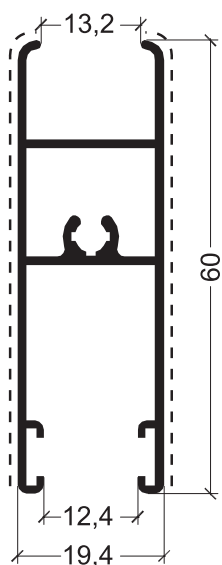
ALBR-352 ZÓCALO/CABEZAL HOJA CORTE A 90° 0,593 kg/m Tiras por Paquete 6
