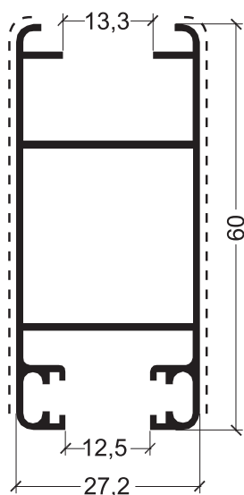
ALBR-353 PARANTE LATERAL HOJA CORTE A 90° 0,645 kg/m Tiras por Paquete 6
