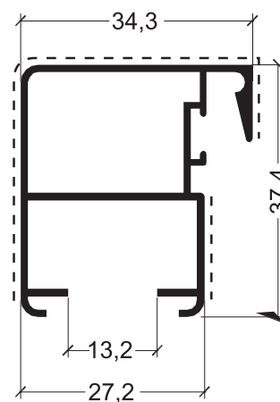
ALBR-354 PARANTE CENTRAL HOJA CORTE A 90° 0,498 kg/m Tiras por Paquete 6
