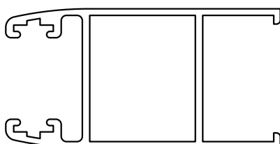
ALBM-248 PARANTE LATERAL HOJA DVH VENTANA Y PUERTA CORREDIZA 0,621 Kg/m Tiras por Paquete 6
