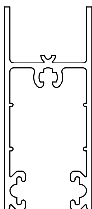
ALBM-249 ZÓCALO Y CABEZAL HOJA DVH VENTANA Y PUERTA CORREDIZA 0,689 kg/m Tiras por Paquete 6
