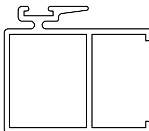
ALBM-250 PARANTE CENTRAL HOJA DVH VENTANA Y PUERTA CORREDIZA 0,583 Kg/m Tiras por Paquete 6
